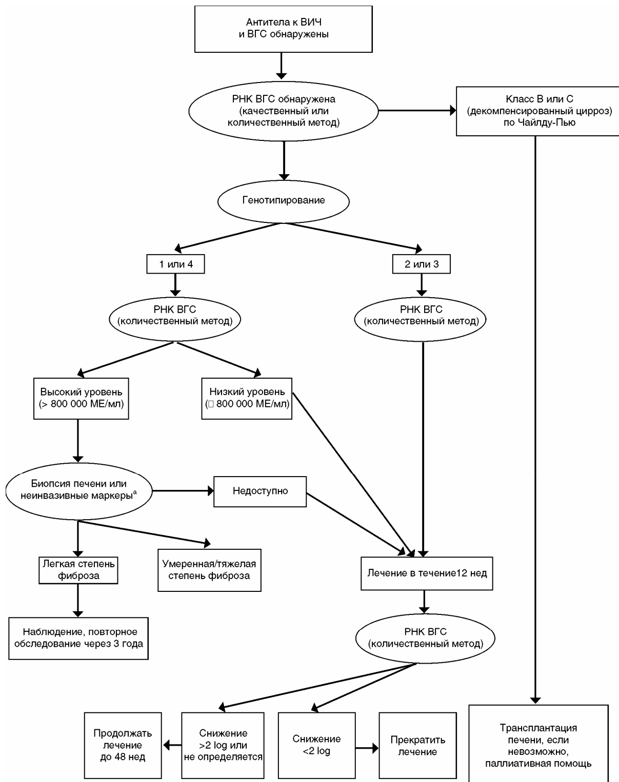
Рис. 6. Алгоритм 1
