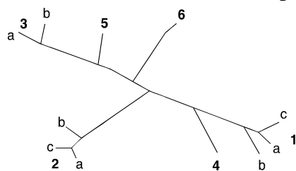
Рис. 4. Филогенетическое древо генотипов и подтипов ВГС
