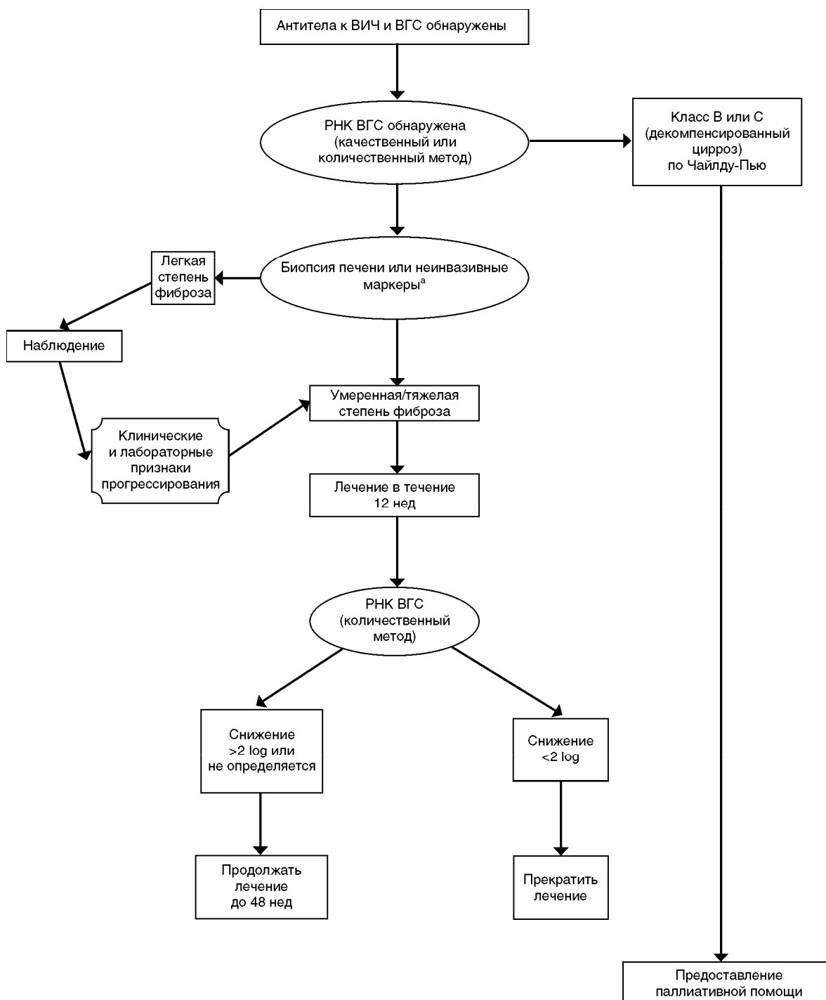
Рис. 7. Алгоритм 2
